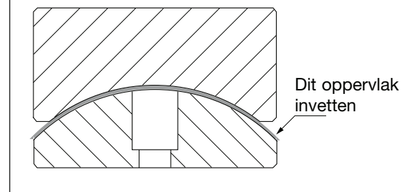
Afbeelding 2 - CAT-zadel
