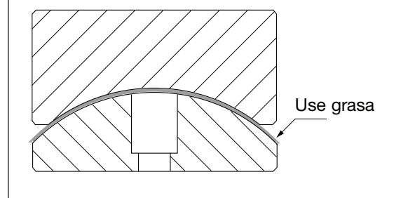
ilustración 2 - asiento orientable CAT
