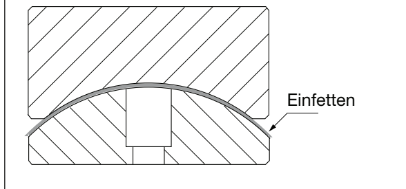
Abbildung 2 - bewegliche CAT-Druckstück
