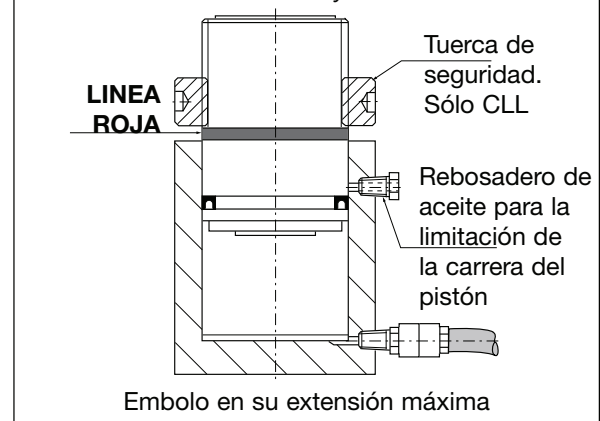
ilustración 1 - Cilindros CLL y CLS
