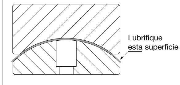
figura 2 - suporte CAT
